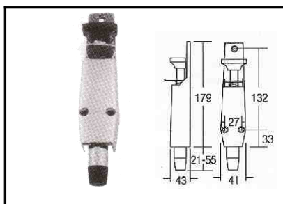
RLSS - DH 031ZA Door Stoper in chrome H 179 x W41mm
